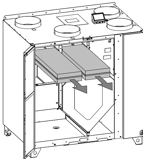
Fig. 4 Changer les filtres
