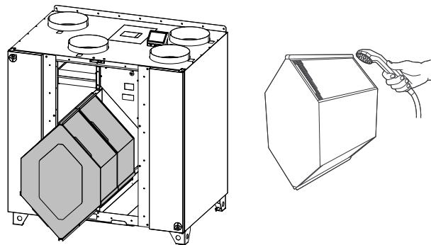
Fig. 5 Démontage et nettoyage de l'échangeur de chaleur
