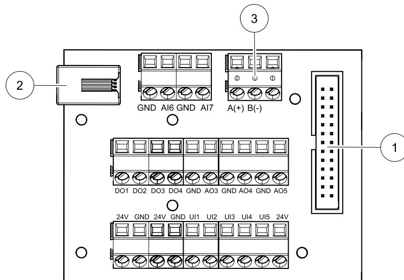
Fig. 7 Carte et boîtier de connexion externe
