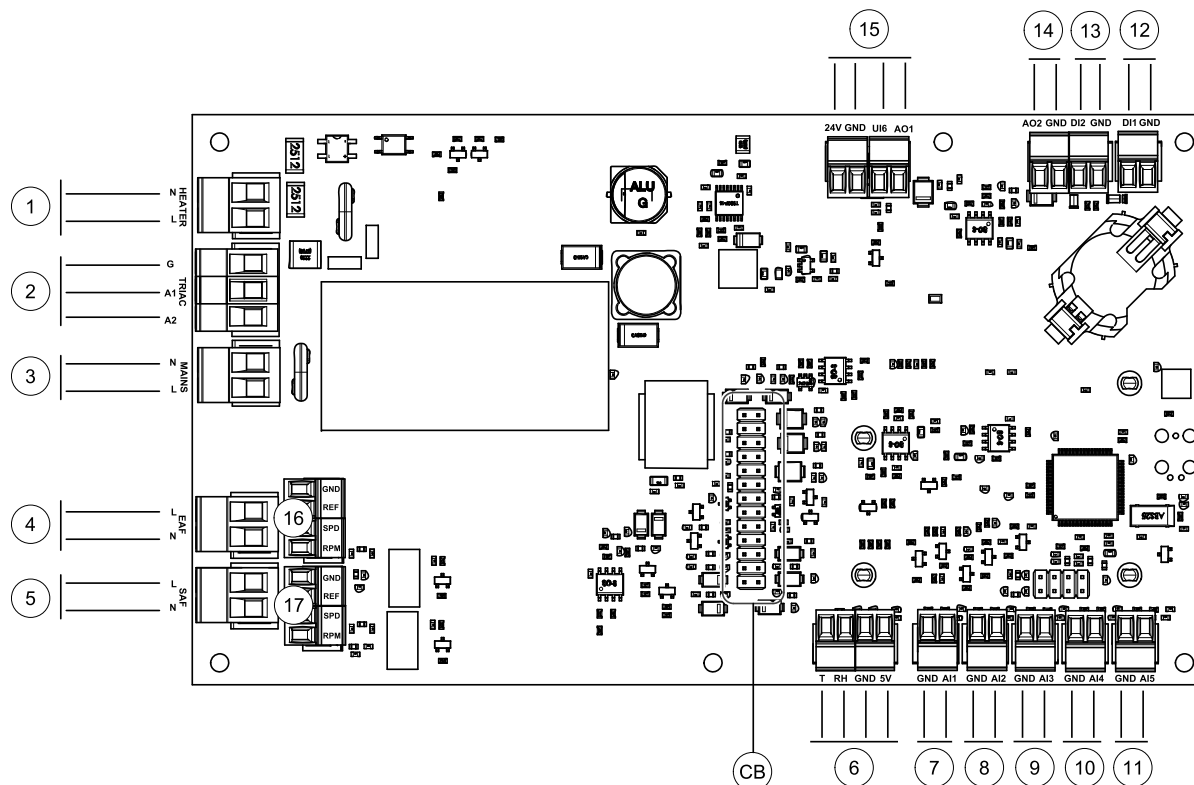
Fig. 6 Raccordements de la carte de régulation
