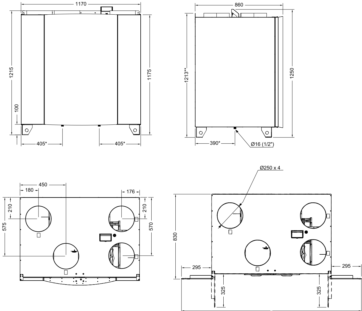
Fig. 2 Dimensions de l'appareil version droite
